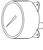
«ФОШ» (по умолчанию) Осевой штуцер с передним фланцем
